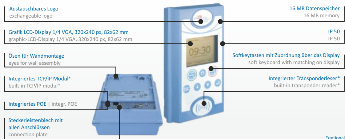
Buchung von Personalzeiten per RFID durch den Mitarbeiter Booking of staff time via RFID by the employer
